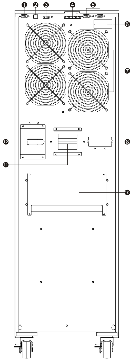
图 2: 30K(L)背板图
