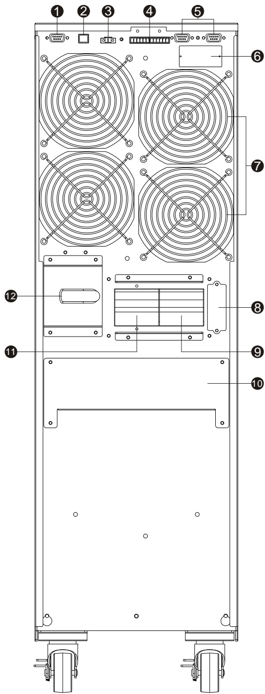
图 1: 10K(L)/15K(L)/20K(L)背板图
