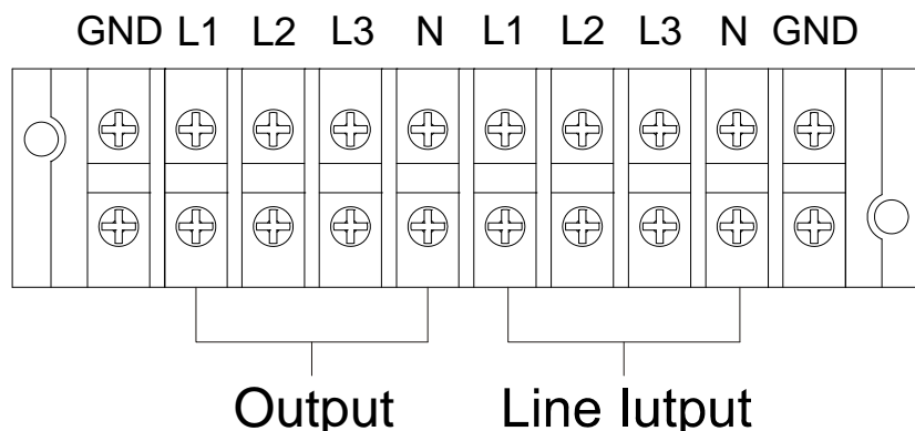
30K (L) 端子布线图
